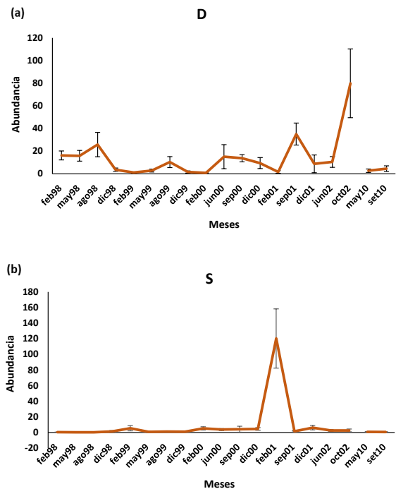
Figura 7. (a) Abundancia del grupo Depredador (D) y (b) Abundancia del grupo Saprófago (S), entre febrero de 1998 y febrero de 2001, mayo y septiembre de 2010.
